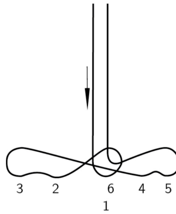
Der Sechsertakt
