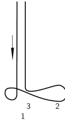
Der Dreiertakt
